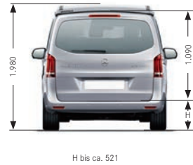
Heck
