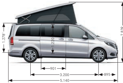
Seitenansicht mit geöffnetem Aufstelldach
